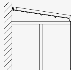
CONTRAVERSA E SOSTEGNO per strutture con profondità da 4,5 a 7,0 m (su richiesta)
