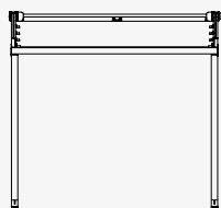
1 CAMPATA L = fino a 450 cm
